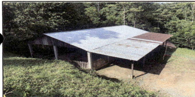
Foto 11: Lamina en mal estado por corrosión
